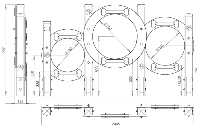
ROZMEROVÝ NÁČRT
